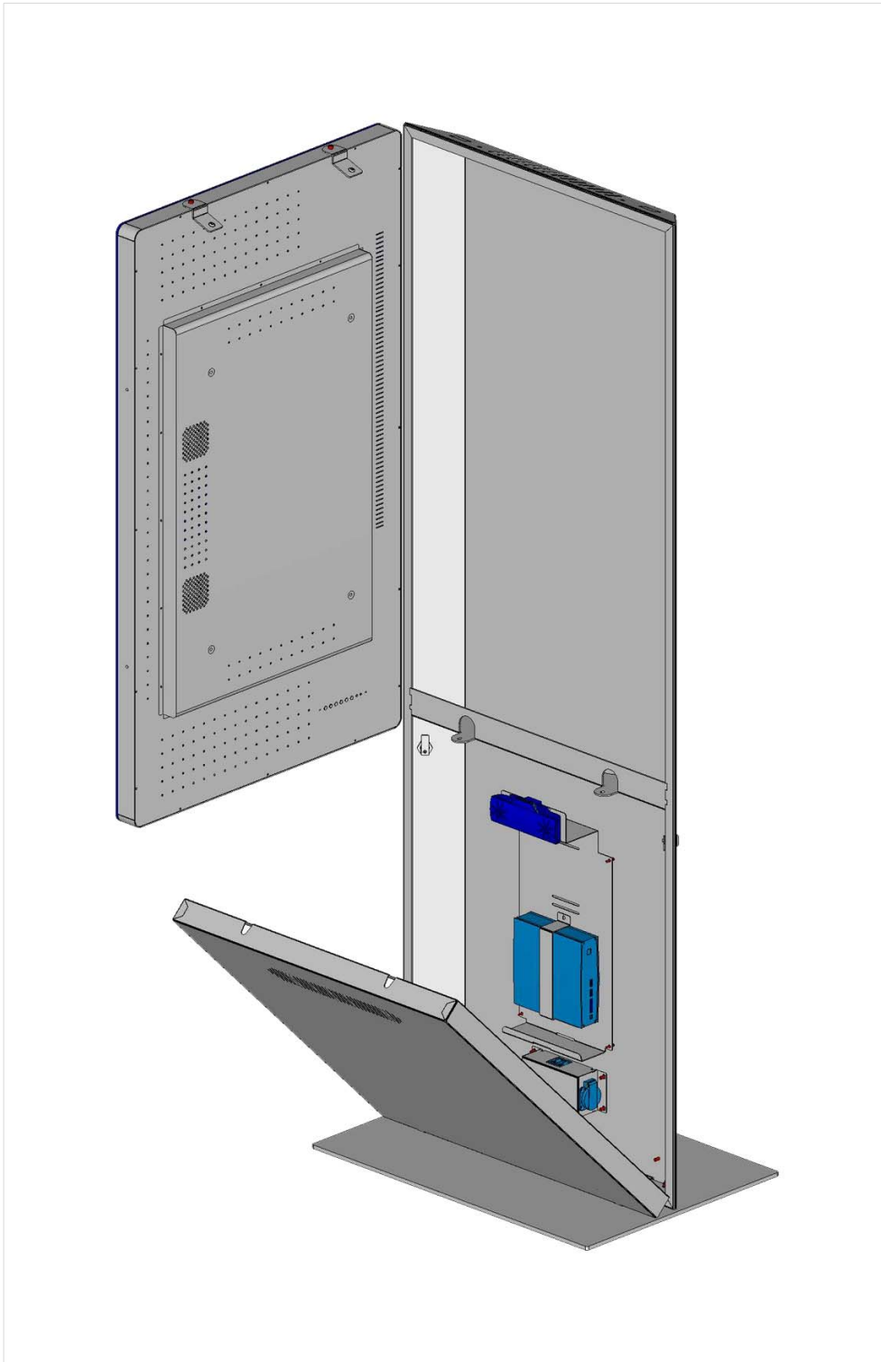
WS-DS Stele - technische Skizze: Gehäuse, Display und Frontklappe
